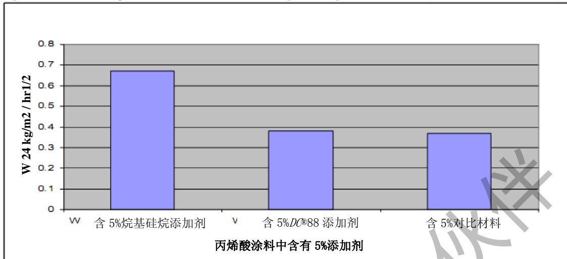
图 1: 道康宁® 88 添加剂有助于减少多孔基材的吸水量 (DIN 标准测试 52617)
